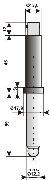
Čidlo pH 521-BNC
