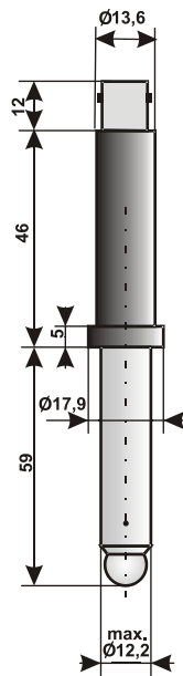
PH SENSOR 521-BNC
