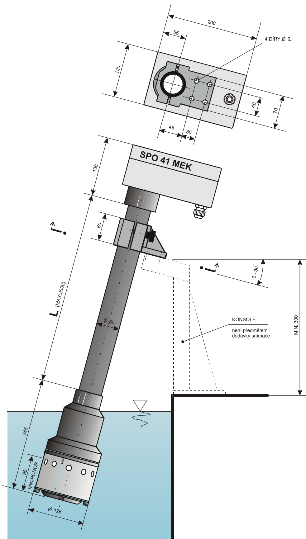
Ponorný snímač SPO 41 MEK
