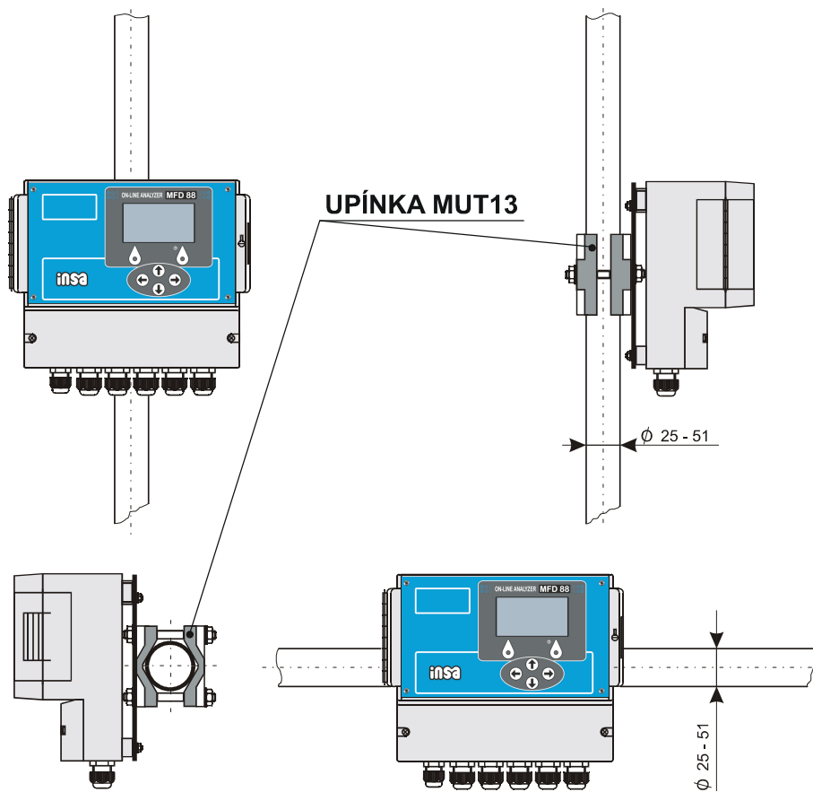
Montáž převodníku řady 88 pomocí upínky MUT 13
