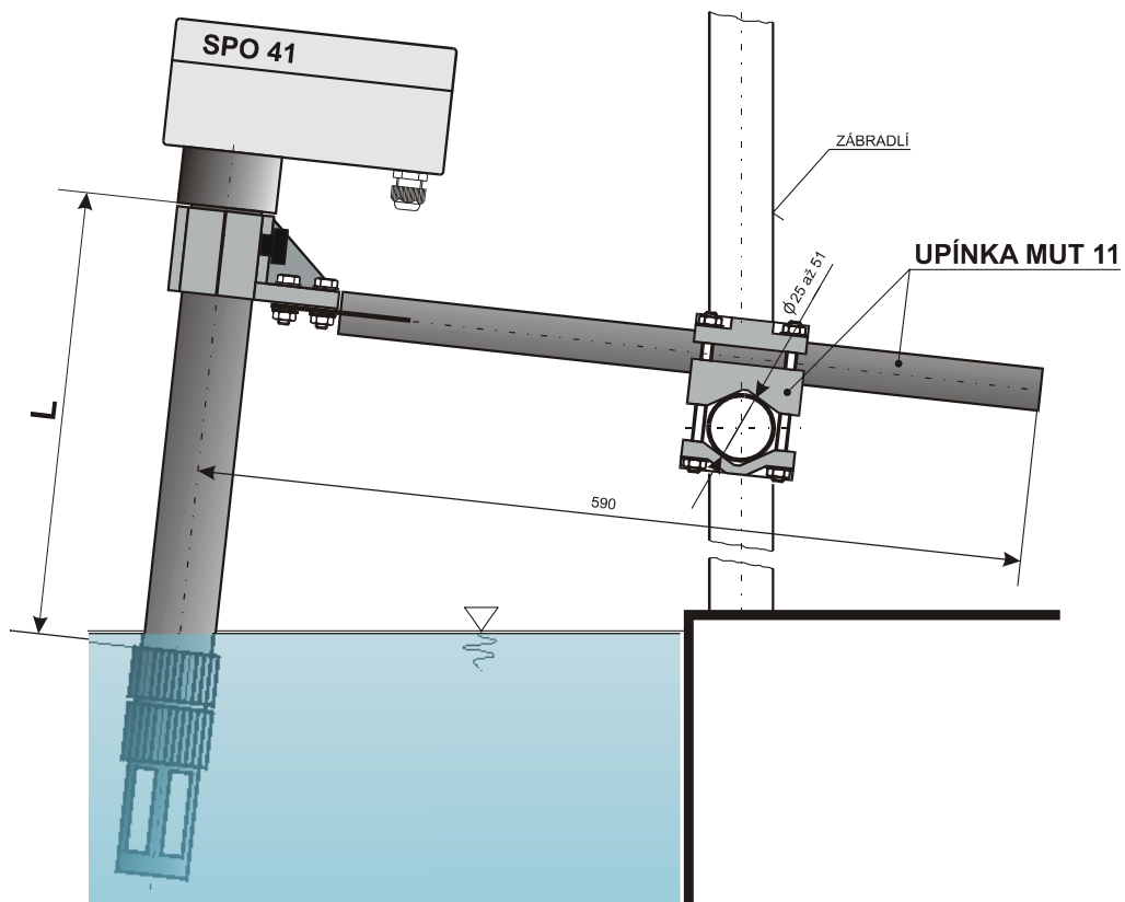
Montáž snímačů SPO pomocí upínky MUT 11
