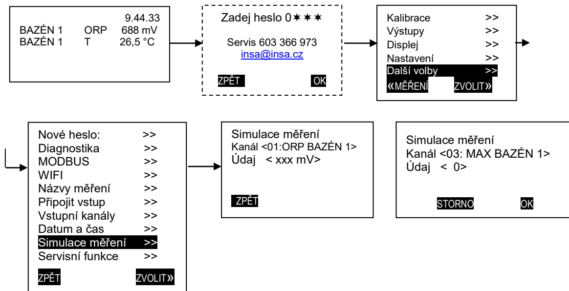
Obr. 13. Simulace měření
